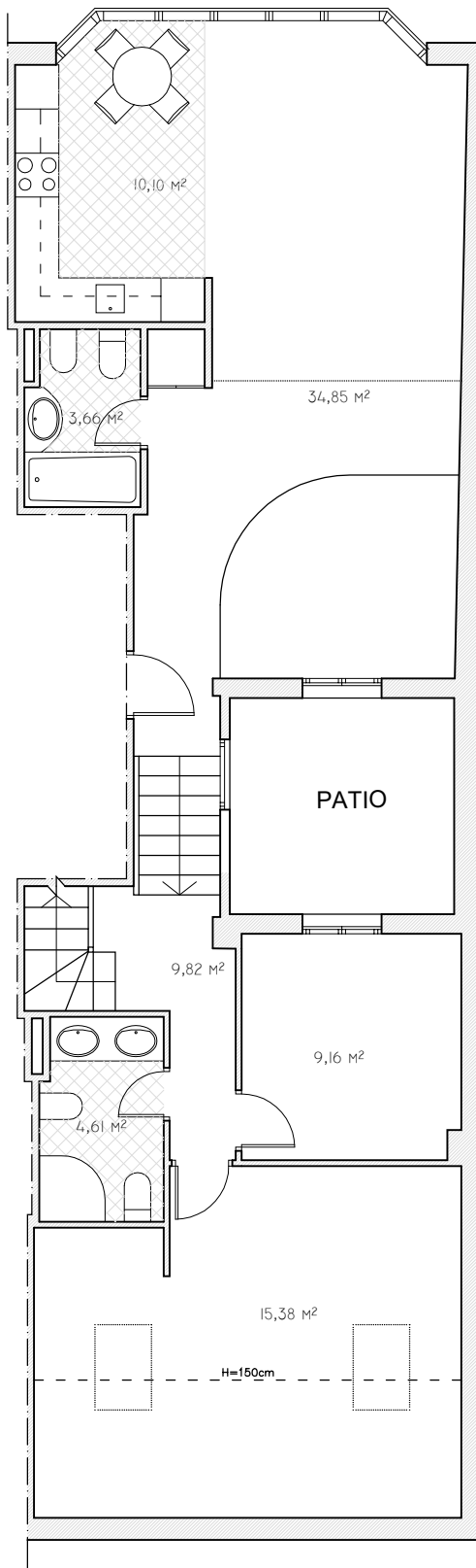
PLANTA 4ª Y ENTREPLANTA SUP. ÚTIL 87,58 m²
